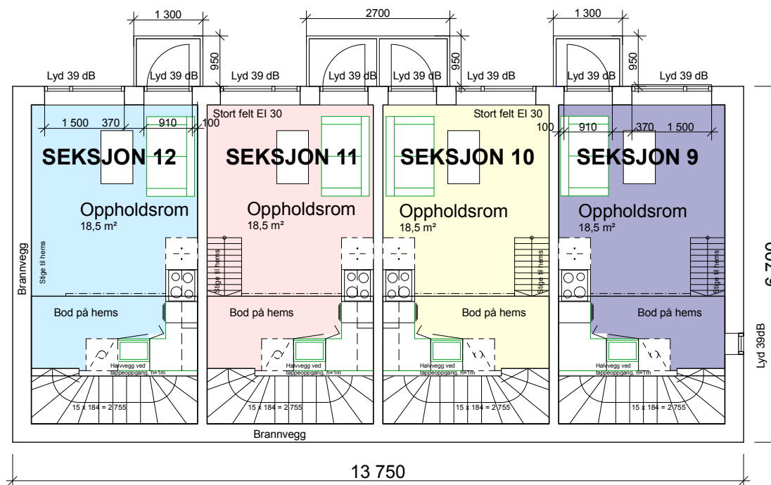
Plan 2. etasje
